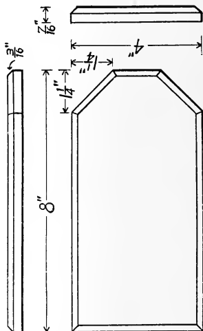
Fig. 275—Match Strike
